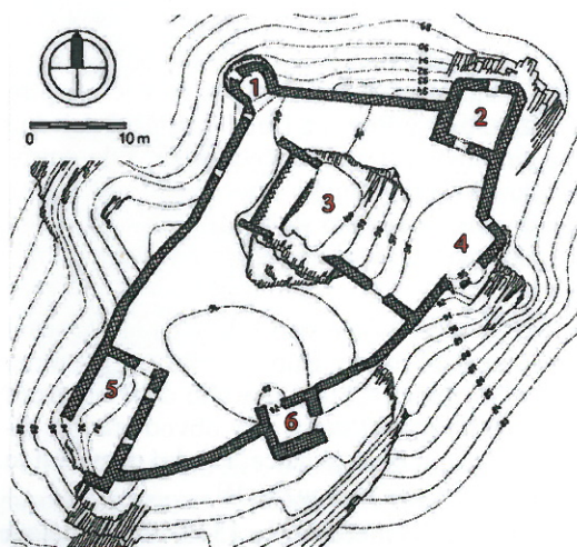
Půdorys hradu podle F. Gabriela a J. Panáčka (zaměření z r. 1992)
